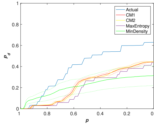
(d) \mathbf{W}^{\mathbf{I}} , \alpha = 0.5
